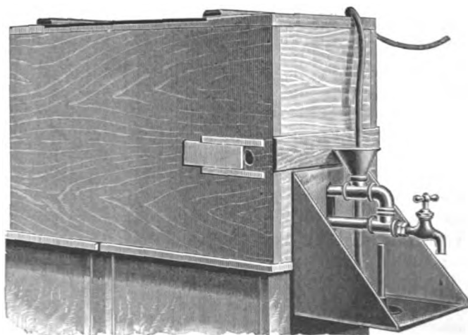
FIG. 1.—Incubator.
